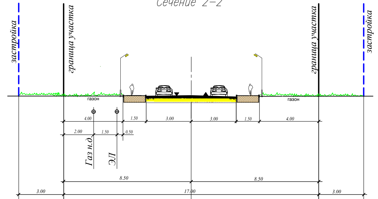
Сечение 2-2
