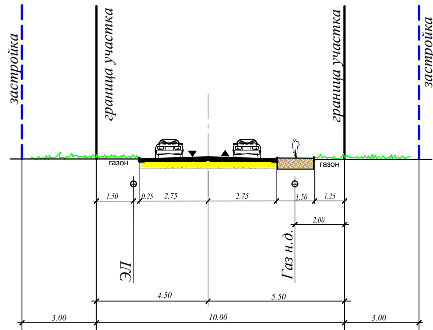
Сечение 1-1
